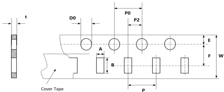
Fig. 5-5 0603 (Paper tape)
