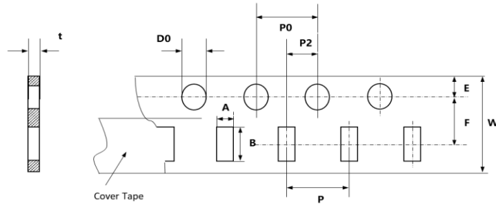
Fig. 5-5 0603 (Paper tape)
