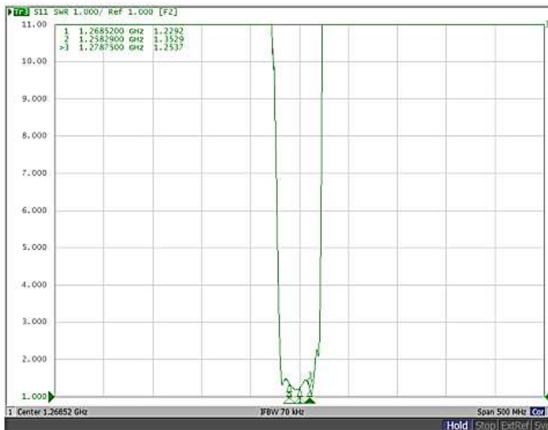
S11 VSWR
