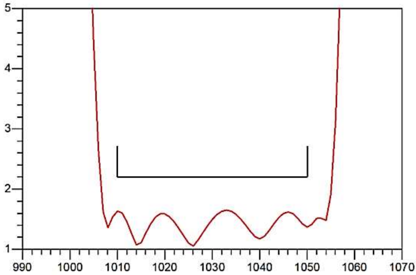
S11 VSWR
