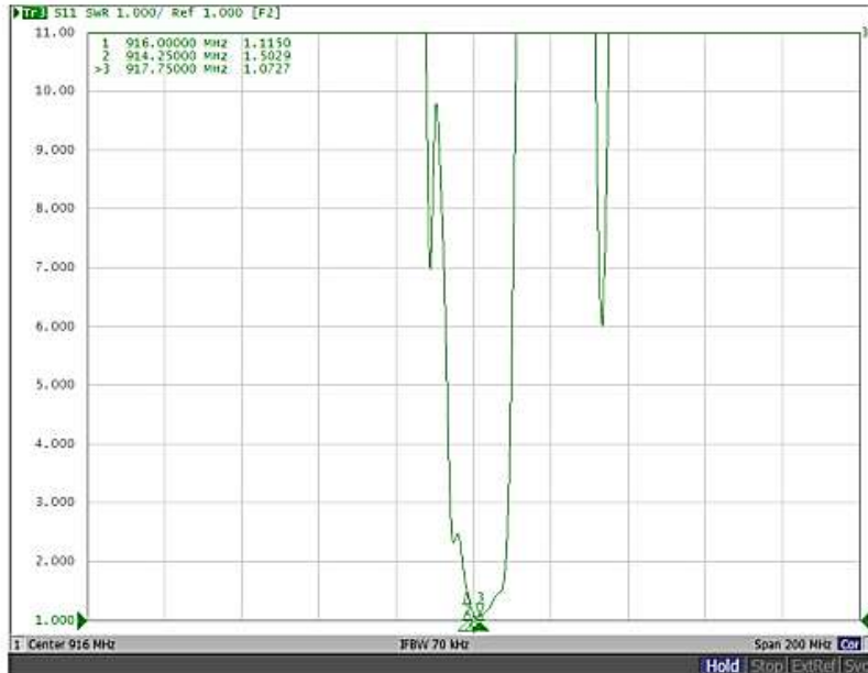
S11 VSWR
